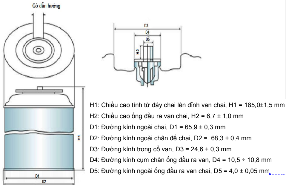
Hình 1. Kích thước chai LPG mini
